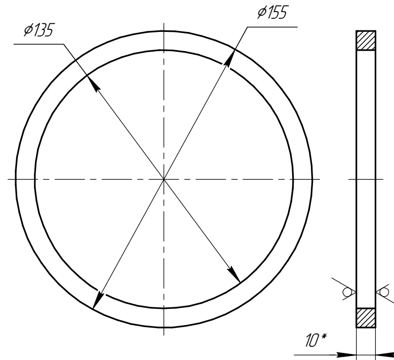
Det. poz. 3
