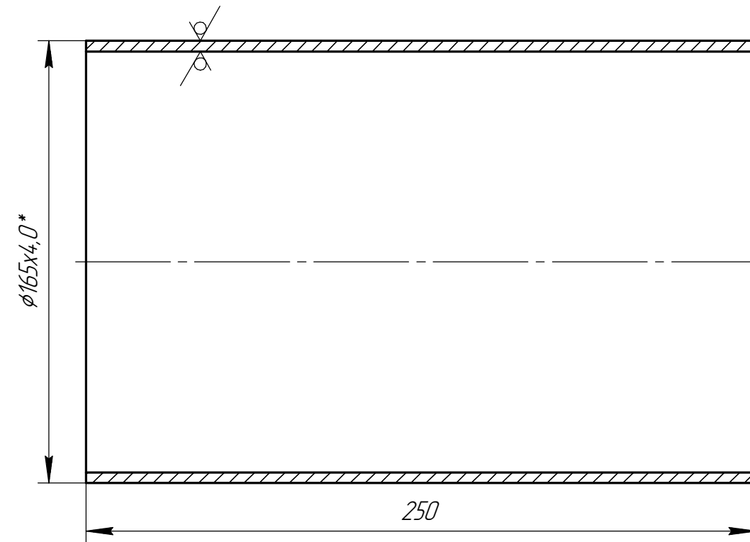
Det. poz. 4
