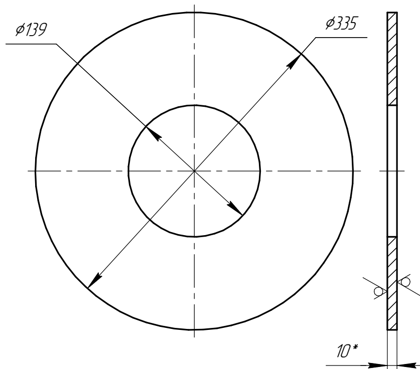
Det. poz. 1 (1:4)
