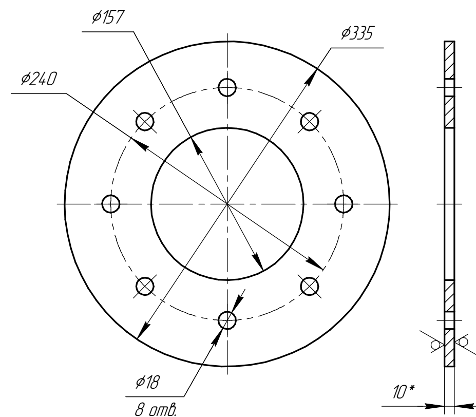
Det. poz. 2 (1:4)
